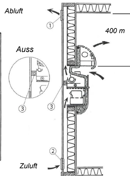
Querschnitt. Siehe Ausschnitt 3
