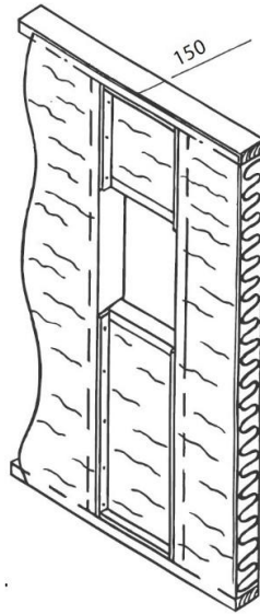
Isolierung 100 mm und Feuchtigkeitsbarriere e
