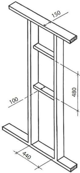
Gerüst 150 mm Ansicht von außen auf den Kühlraum
