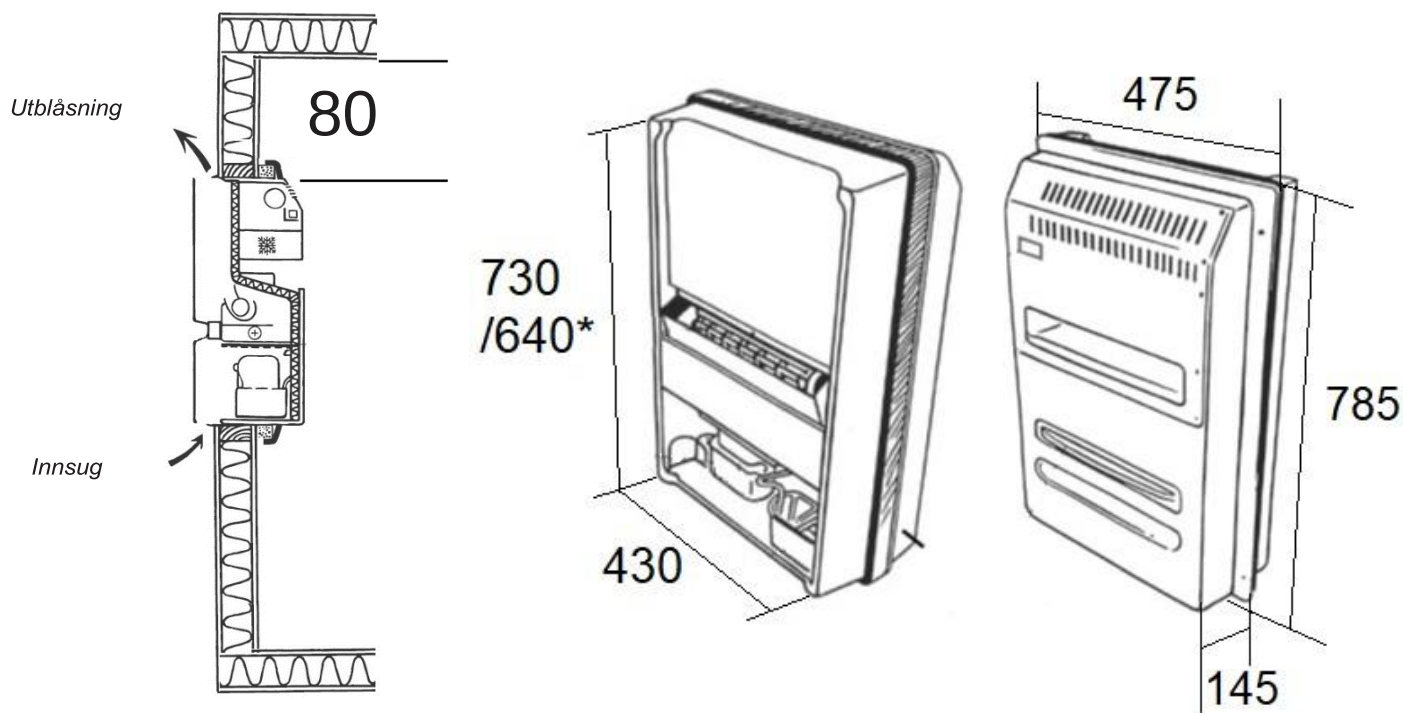
Monteringsalternativ 1 i eksempel bilde Luft ledes igjennom plastdeksel.
