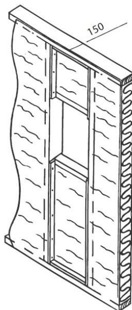
Isolasjon 100mm og fuktspærre Sett fra utsiden av kjølerommet
